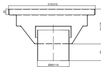
HAUTEUR RÉDUITE
