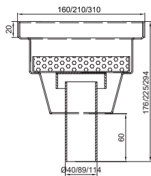
HAUTEUR NORMALE
